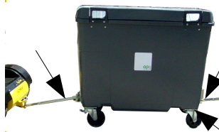
SSATKIT - kit d'attelage complet pour conteneurs à 4 roues
