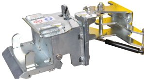
CSATTPIR - Attelage semi-automatique Piranha pour tubes carrés
