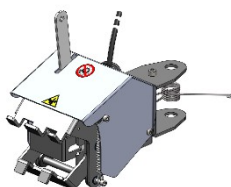
CSATT02 - Attelage semi-automatique CROCO pour tube. Charge maxi : 3500kg
